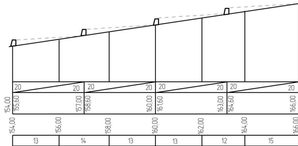
Продольный профиль оврага с барражами
