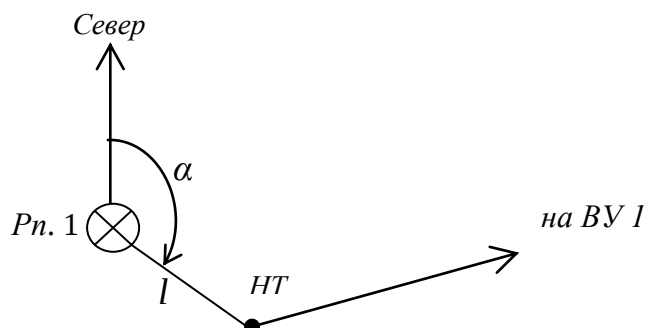
Рисунок 3.12 – Схема привязки точки трассы к временному реперу (ситуационному объекту)
