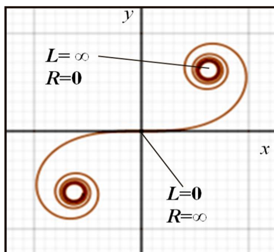
Рисунок 3.6 – График клотоиды
