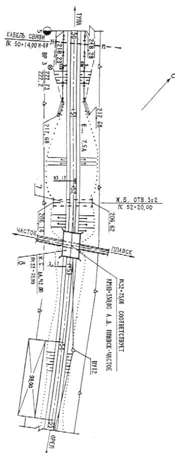
Рисунок 3.10 - Пример выполнения плана автомобильной дороги общего пользования при масштабе 1:2000 и крупнее
