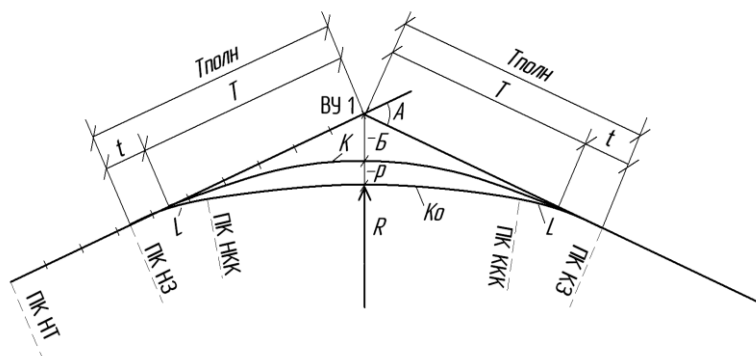
Рис. 3.7. Схема вписывания круговой кривой с переходными кривыми
