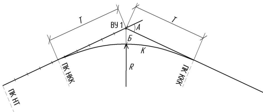
Рис. 3.5. Схема вписывания круговой кривой без переход-
