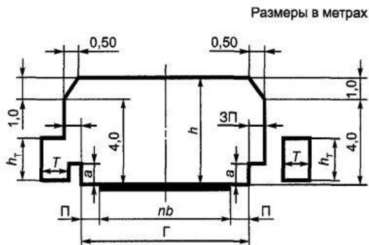
a - при отсутствии разделительной полосы
