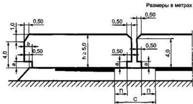
Рисунок 3 - Схемы габаритов приближения конструкций под путепроводами
