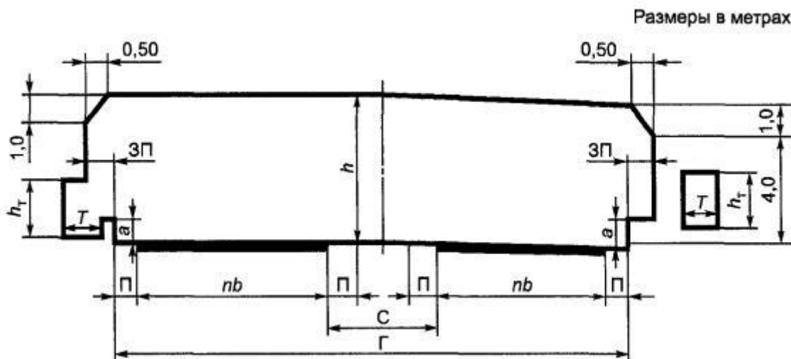
б - с разделительной полосой без ограждений
